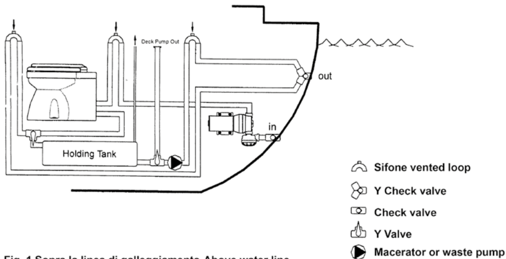
Fig. 1 Sopra la linea di galleggiamento-Above water line
