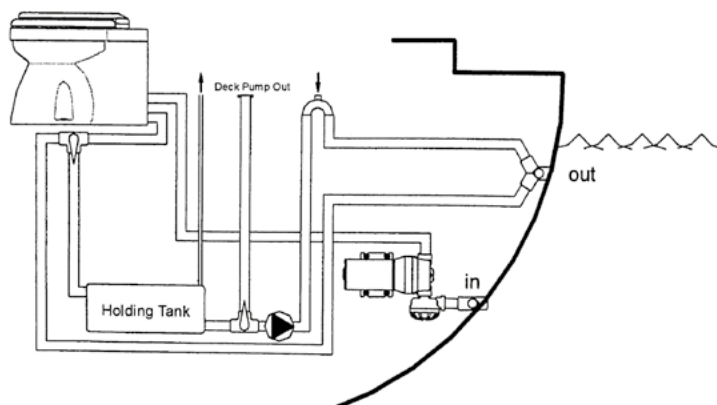
Fig. 1 Sopra la linea di galleggiamento-Above water line
